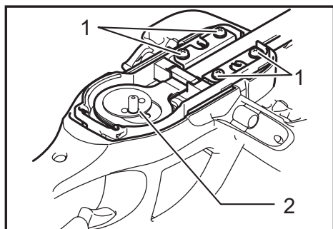
► 1. Vis 2. Rondelle
