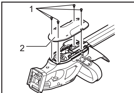
► 1. Vis 2. Sous-couvercle
