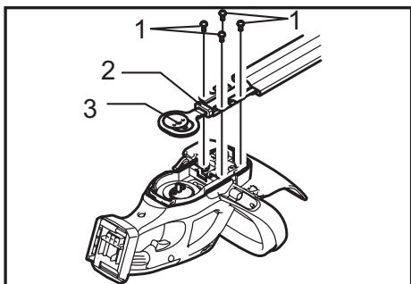
► 1. Vis 2. Éponge 3. Rondelle
