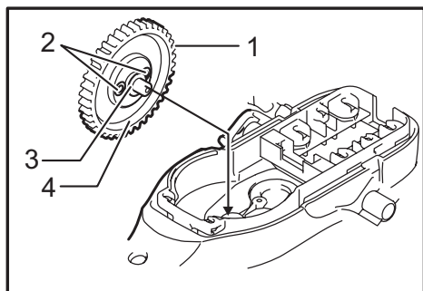
► 1. Motor 2. Fundas 3. Arandela 4. Ranura
