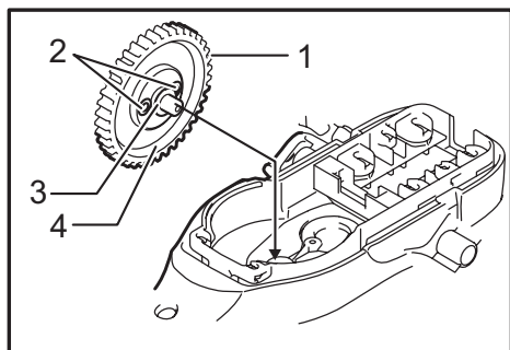
► 1. Engrenage 2. Manchons 3. Rondelle 4. Rainure
