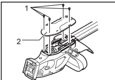
► 1. Tornillos 2. Cubierta por debajo
