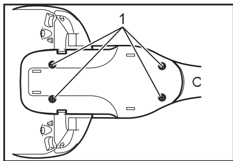
► 1. Screws
