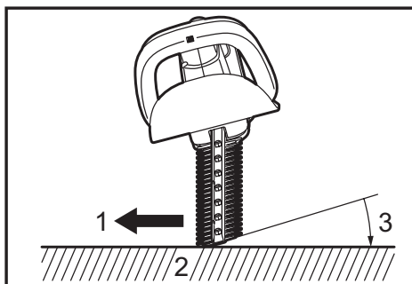
► 1. Dirección de podado 2. Superficie del seto a ser podada 3. Inclinación de las cuchillas
