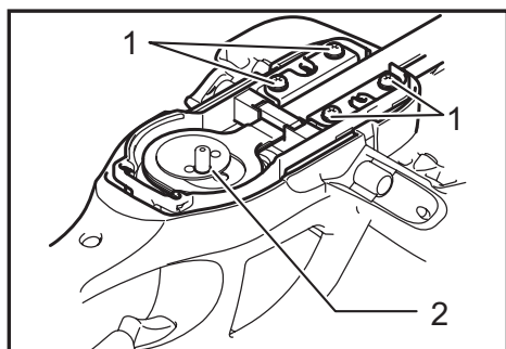
► 1. Tornillos 2. Arandela
